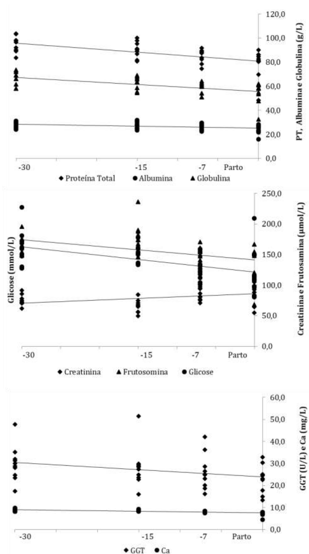
Fig.1. Representação gráfica da dinâmica de metabólitos do sangue de cabras da raça Moxotó nos períodos do pré-parto (-30, -15, -7 dias) e Parto.
